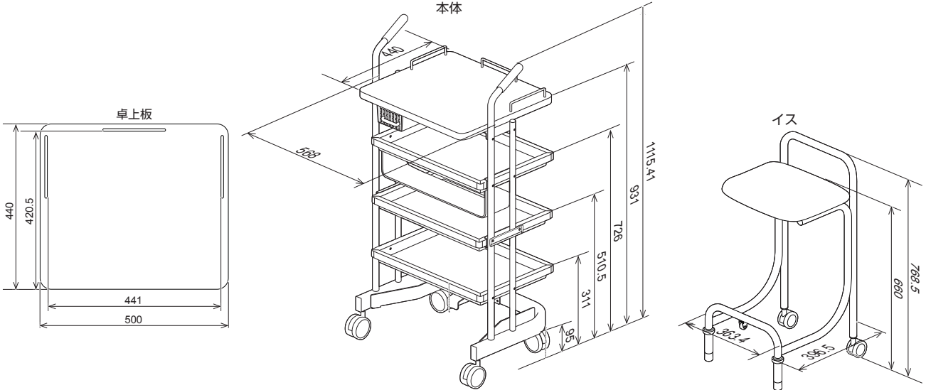
寸法図 (mm)
