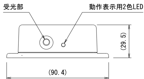
赤外線式ワイヤレス受光器 S=1/2
