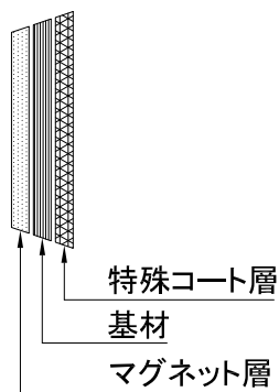
WOLスクリーン構造図
