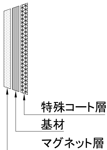
WOLスクリーン構造図
